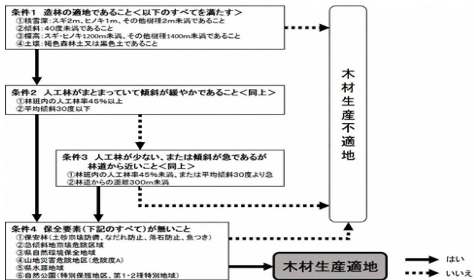
図Ⅱ-5-2-1 木材生産適地の抽出条件および手順
