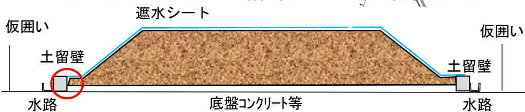
底盤コンクリート詳細図
