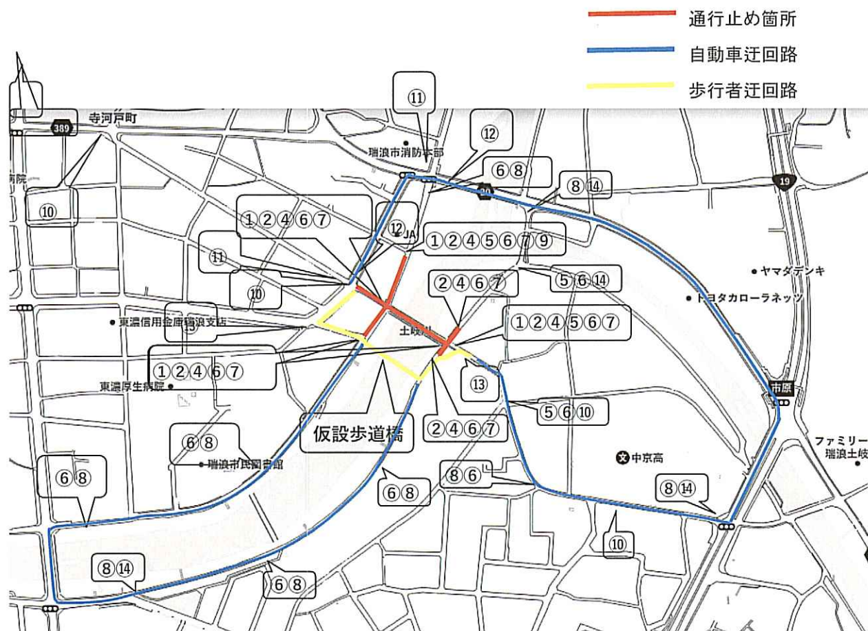
安全施設設置位置図
