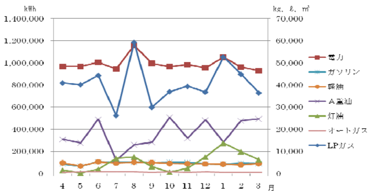
グラフ1. 燃料等の使用量
