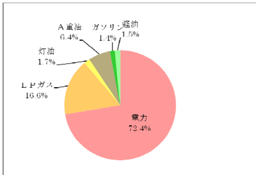
グラフ3. 燃料等の種別の二酸化炭素排出割合
