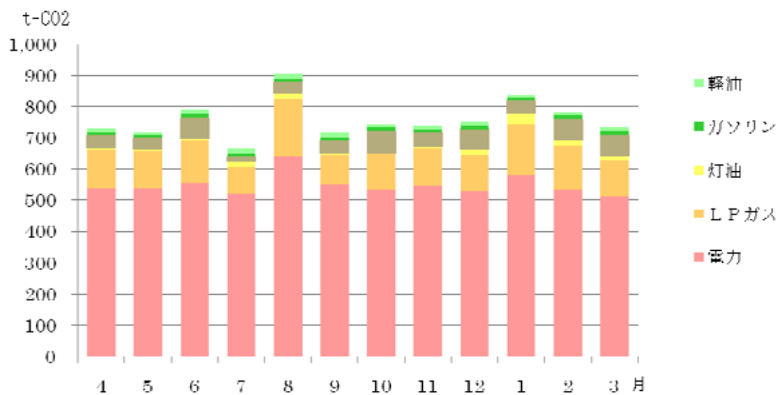
グラフ2. 燃料等の種別の二酸化炭素排出量
