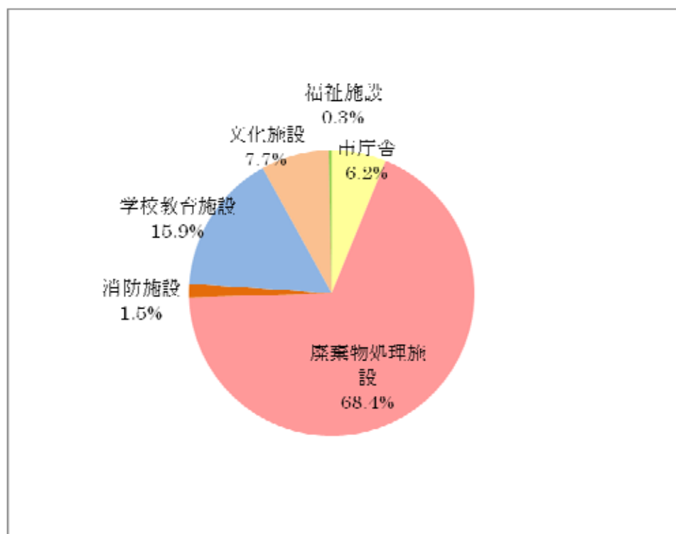
グラフ 5. 分野別のエネルギー起源二酸化炭素排出割合
