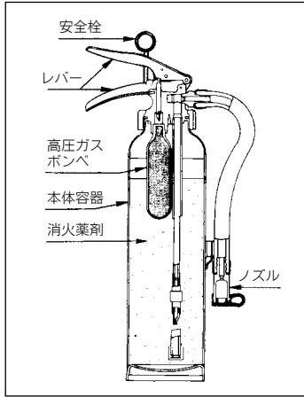
図一 加圧式粉末消火器断面図
