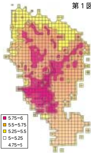
複合地震による瑞浪市の想定震度分布
