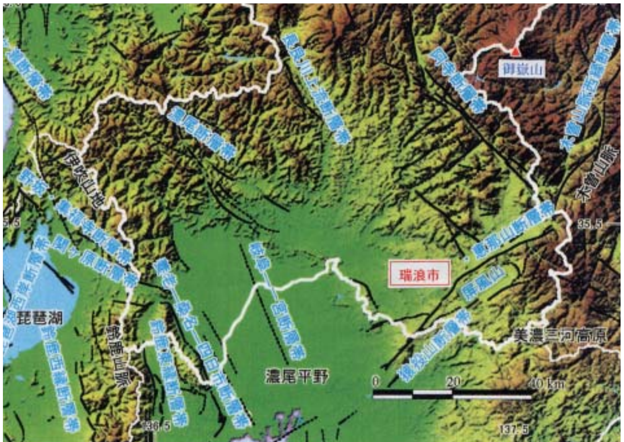
▲ 岐阜県南部の活断層(日本の地震活動より)
