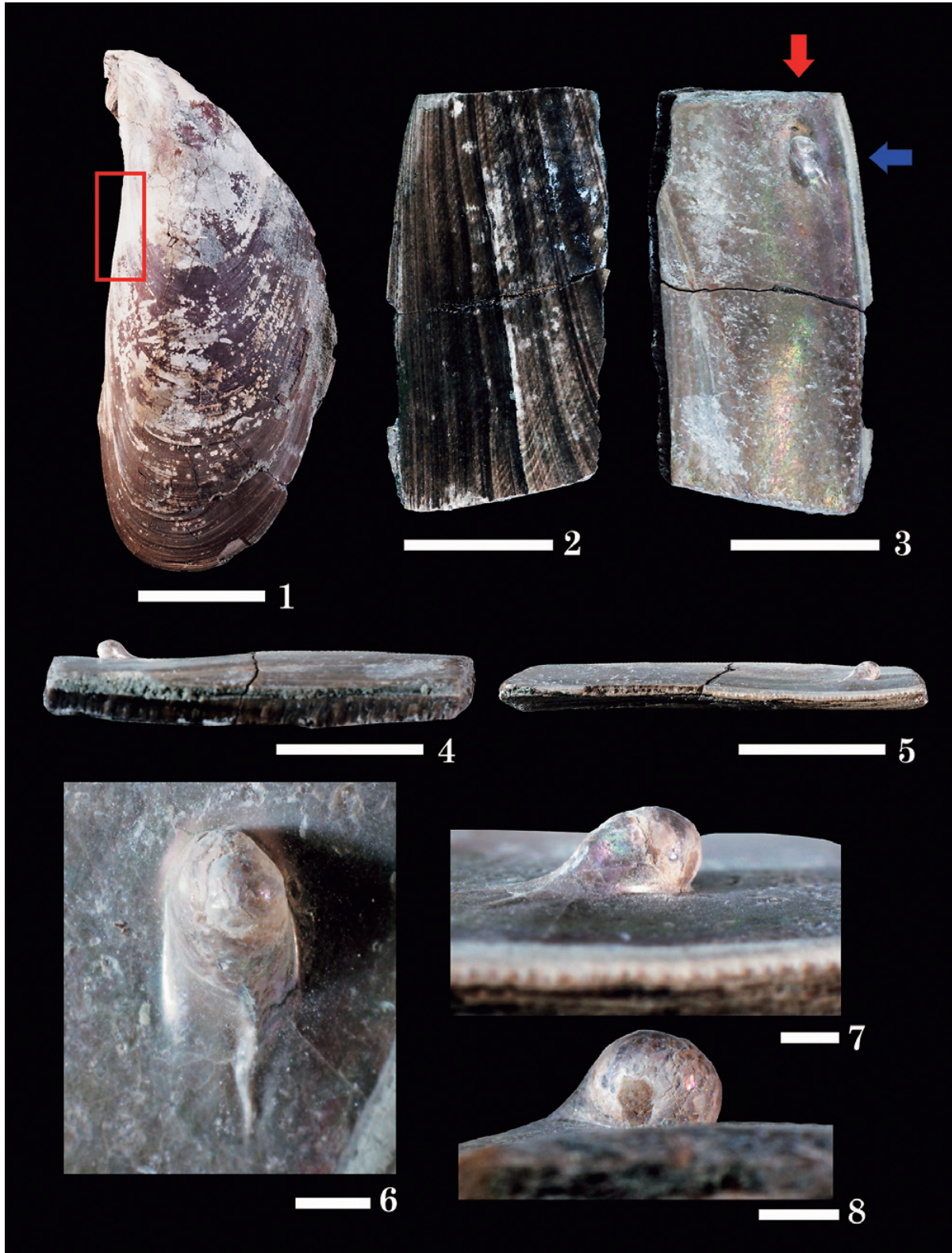
図 1. Crenomytilus grayanus と付着する真珠化石. 1. Crenomytilus grayanus , MFM16002. 赤枠は MFM16023 と推定される部位. 2-5. 真珠化石とその母貝 C. grayanus , MFM16023. 2, C. grayanus の殻表; 3, C. grayanus の内面, 赤および青矢印は, 図 1.7 と図 1.8 の撮影位置と方向; 4, 左側面; 5, 右側面. 6-8. 真珠化石. 6, 上面から撮影; 7, 青矢印より撮影; 8, 赤矢印より撮影. 1 のスケールは 3.0 cm, 2-5 のスケールは 1.0 cm, 6-8 のスケールは 1.0 mm.
