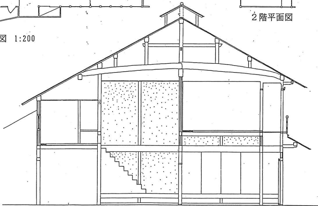
断面図 1:100
