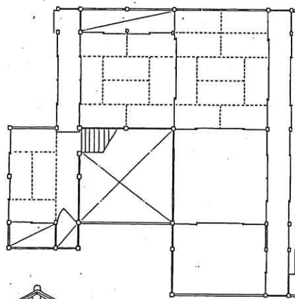
2階平面図
